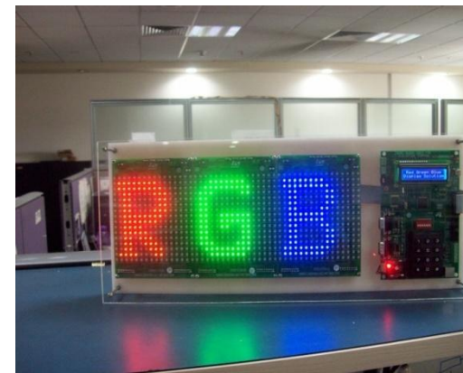
STEVAL-ILL032V1*
