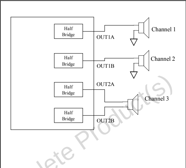
Figure 30. OCFG = 01
