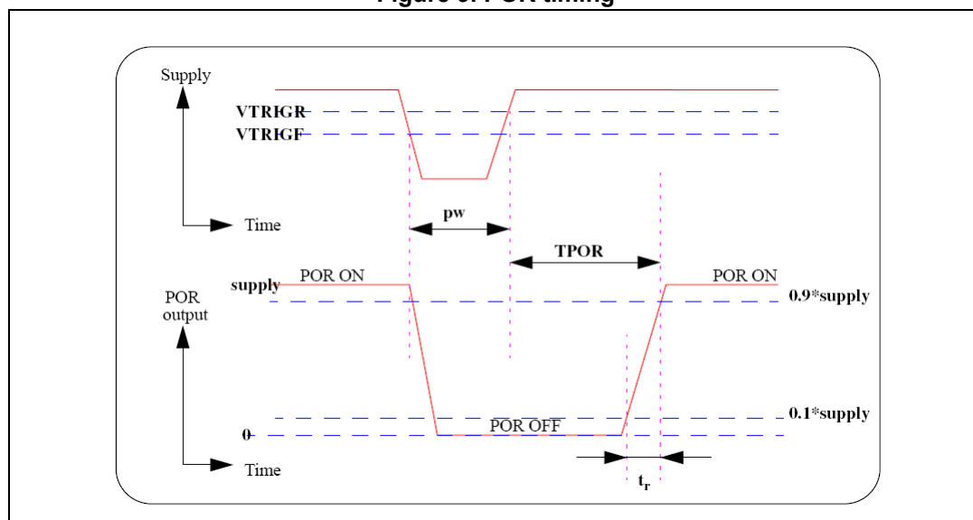
Figure 9. POR timing
