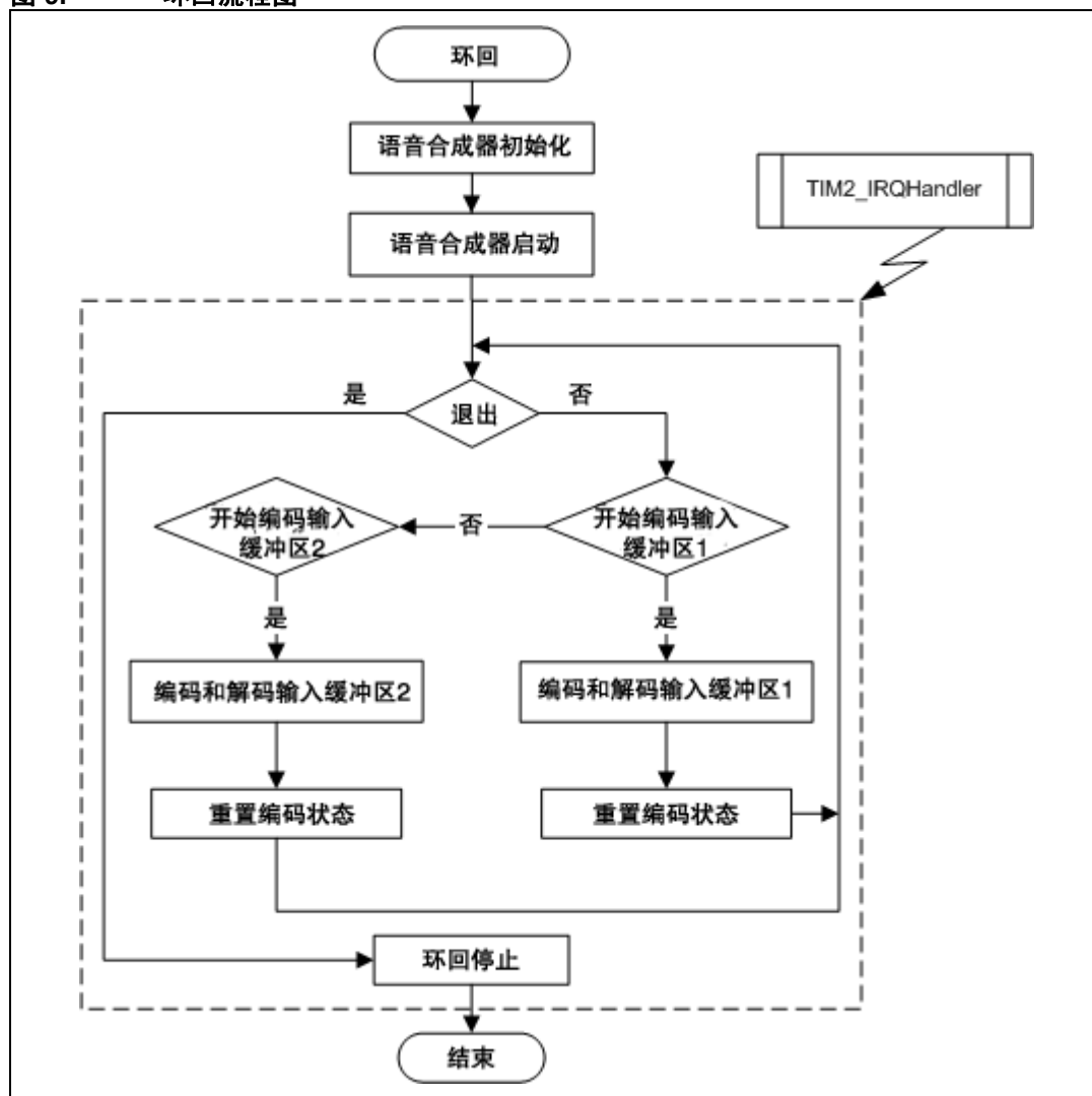
图 9. 环回流程图
