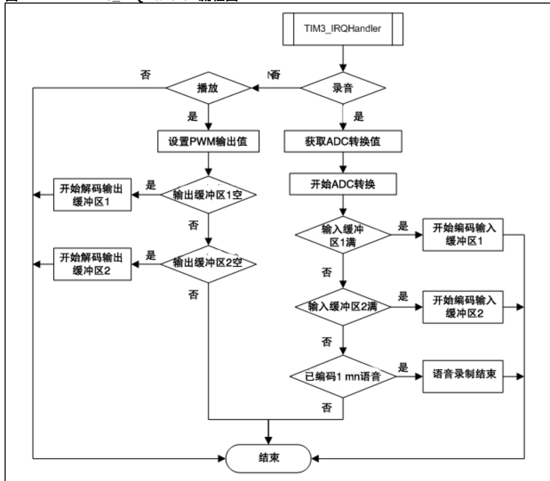
图 7. TIM3_IRQHandler 流程图
