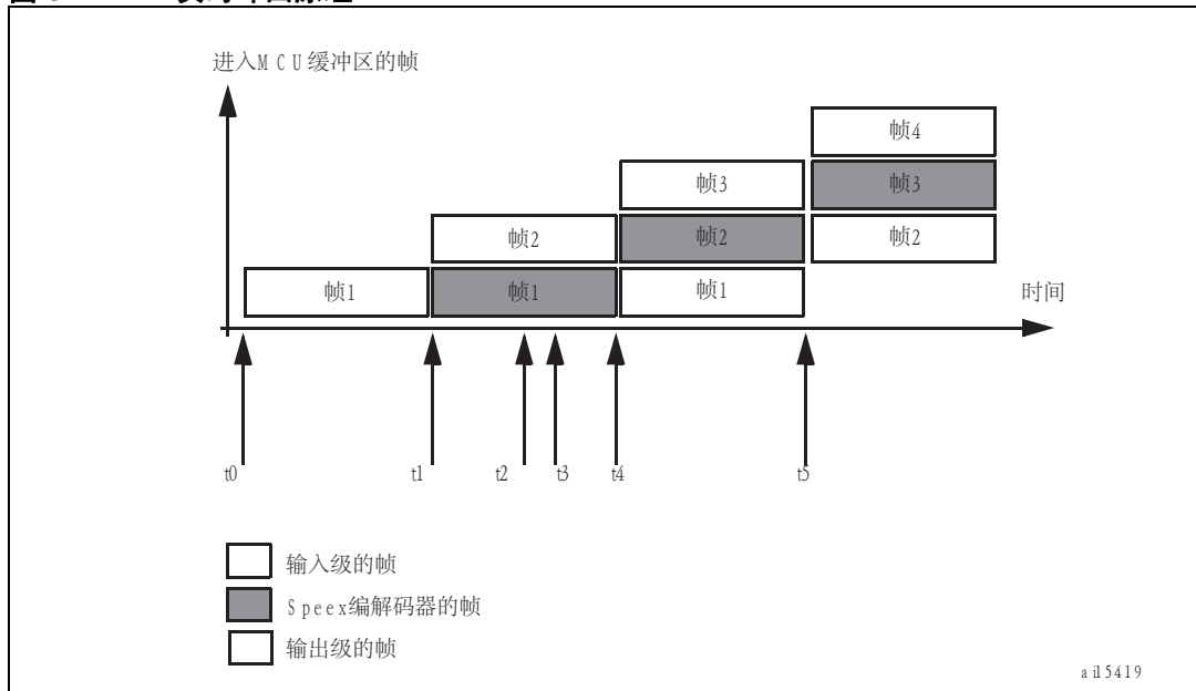
图 8. 实时环回原理
