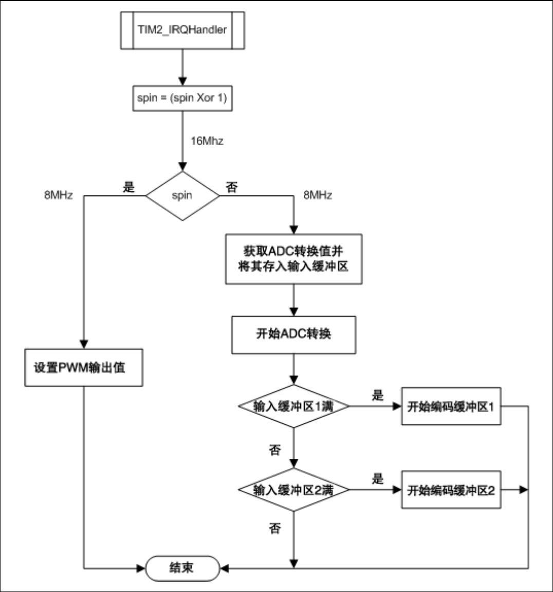
图 10. TIM2_IRQHandler 流程图
