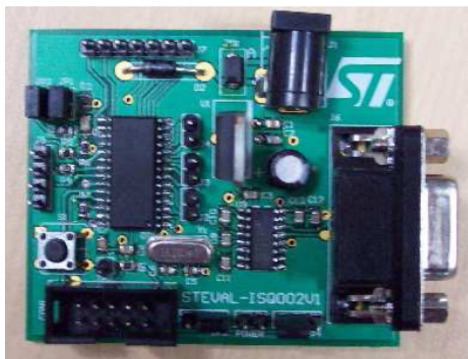
Figure 29. STEVAL-ISQ002V1
