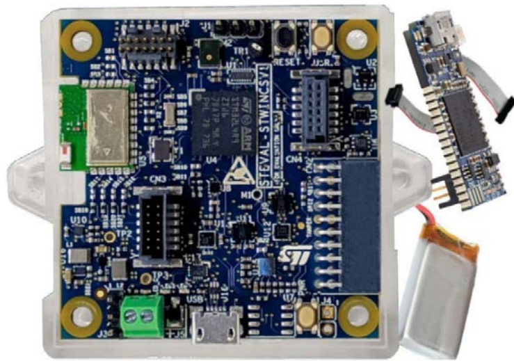
STEVAL-STWINKT1
