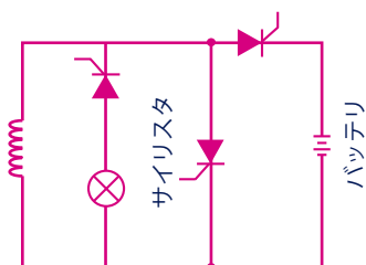
単相ブリッジ シリーズ + シャント・サイリスタ
