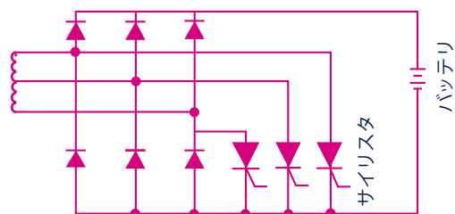
3相ブリッジ シャント・サイリスタ
