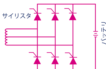
3相ブリッジ シリーズ・サイリスタ
