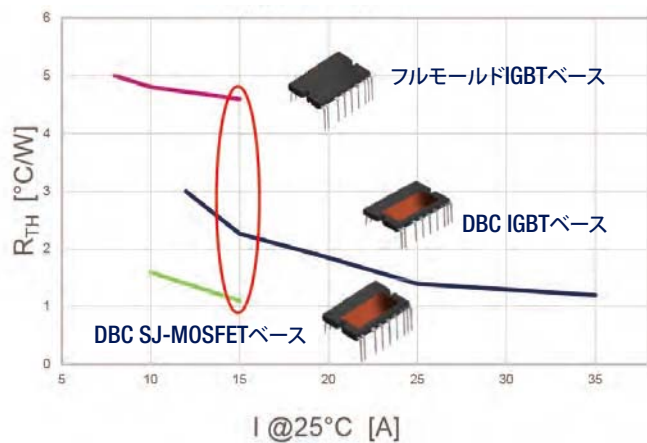
図1: 低 R_{TH} 値
