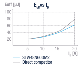
ターンオフ・エネルギー ( E_{off} vs I_D ) @ V_{DD} = 400V , V_{GS} = 10V \div 0V , ダイオード = 2006 SiC, R_G = 4.7 \Omega
