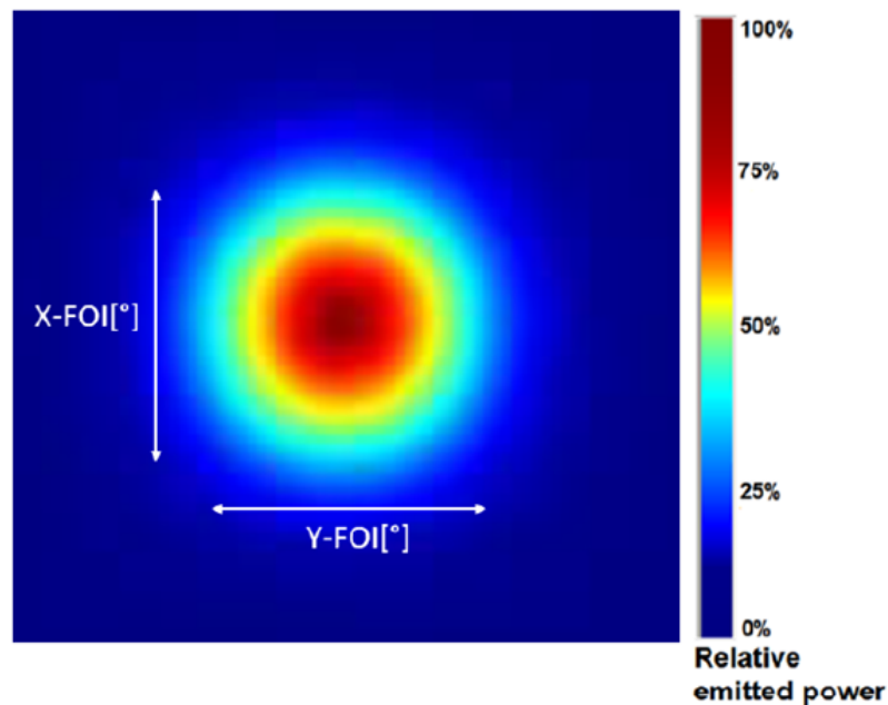
Figure 5. Example of the VL53L4CD FoI
