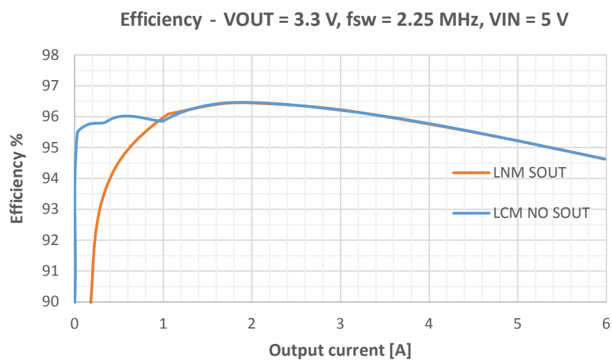
Figure 30. Efficiency (lin. scale)
