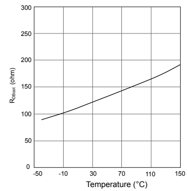
Figure 12. Typ R_{Dboot} vs. T_J
