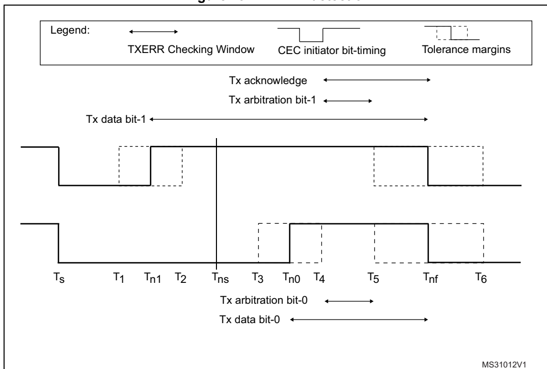
Figure 292. TXERR detection
