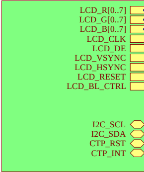
U_MODULE_TO_MAIN_BOARD_CONNECTOR MODULE_TO_MAIN_BOARD_CONNECTOR.SchDoc
