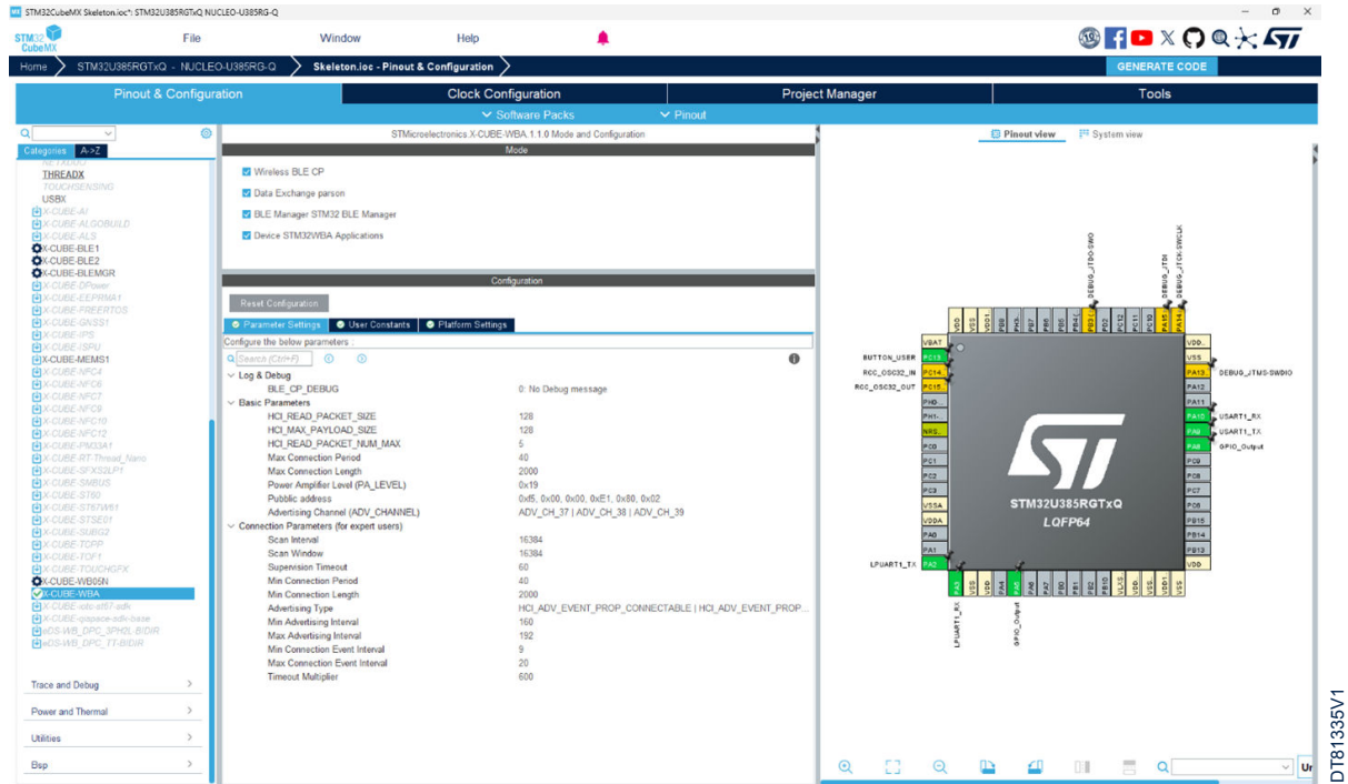
Figure 18. STM32CubeMX - Parameter settings
