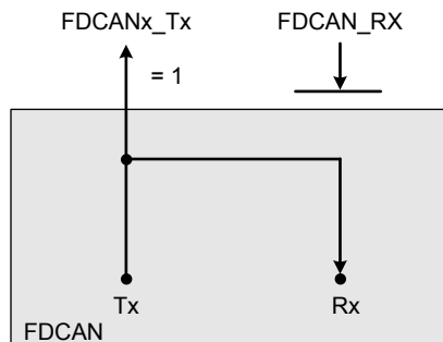
图 22. 外部环回模式下的引脚控制
