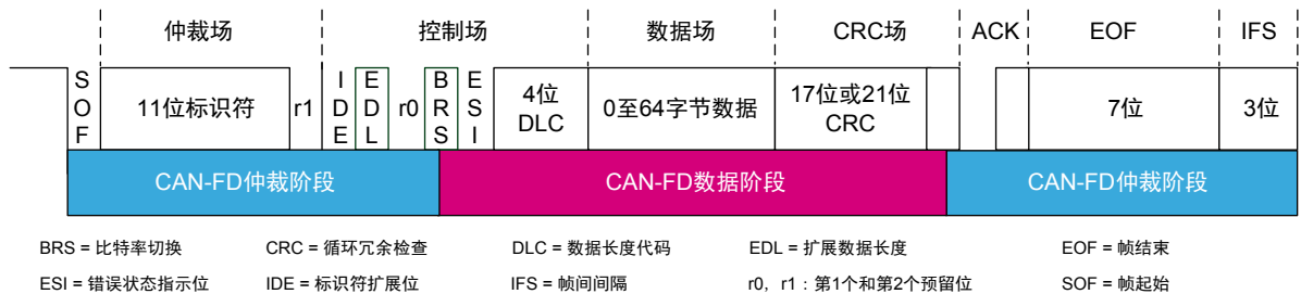
图 1. 标准 CAN-FD 帧
