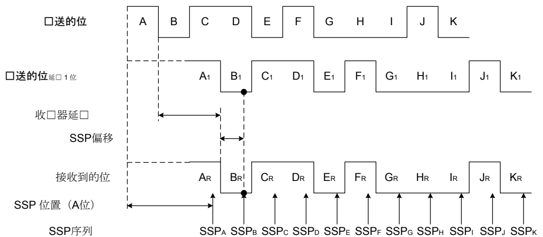
图 26. 发送延迟补偿中的 SSP 位置
