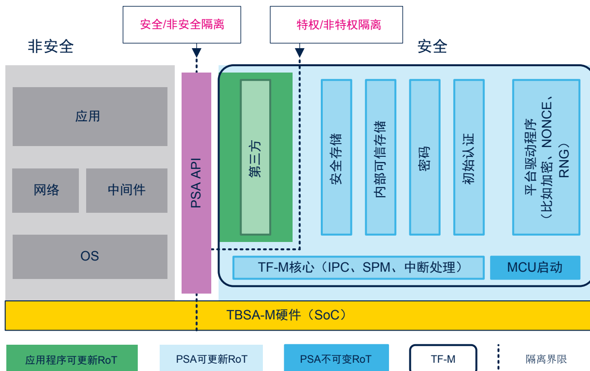
图 1. TF-M 概述
