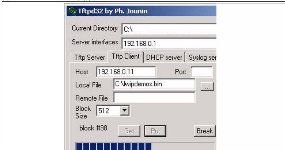
图 4. TFTPD32 对话框
