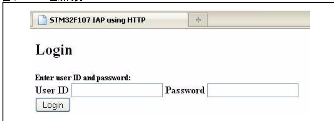
图 8. 登录网页
