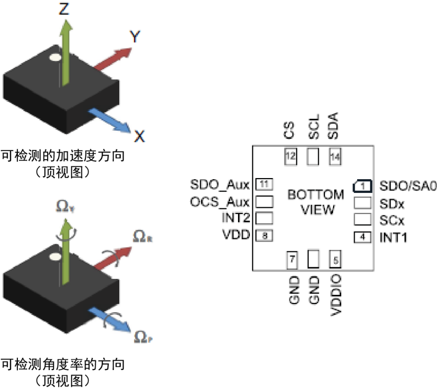
图 1. 引脚连接
