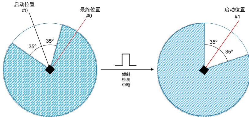
图 23. 倾斜度检测
