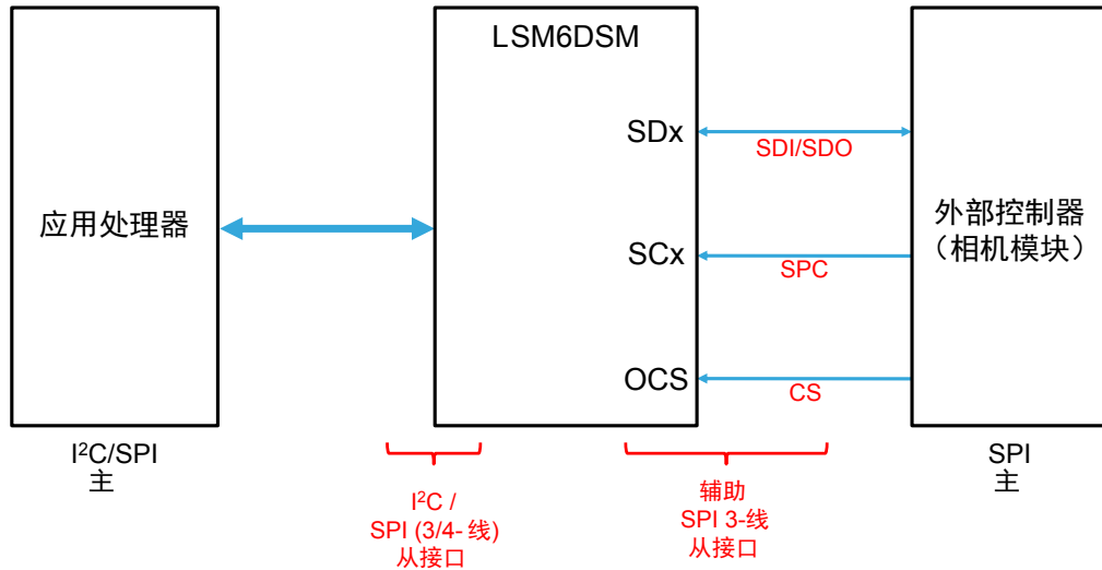
图 30. 模式 3/4 下的外部控制器连接 (SPI 3 线)
