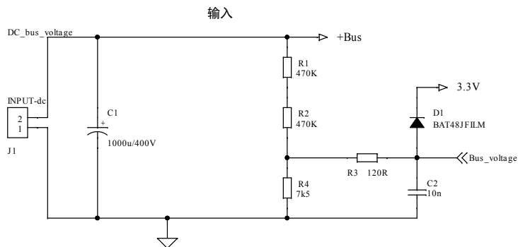
图 1. STEVAL-IPM20B 板原理图 (图 1, 共 5 图)
