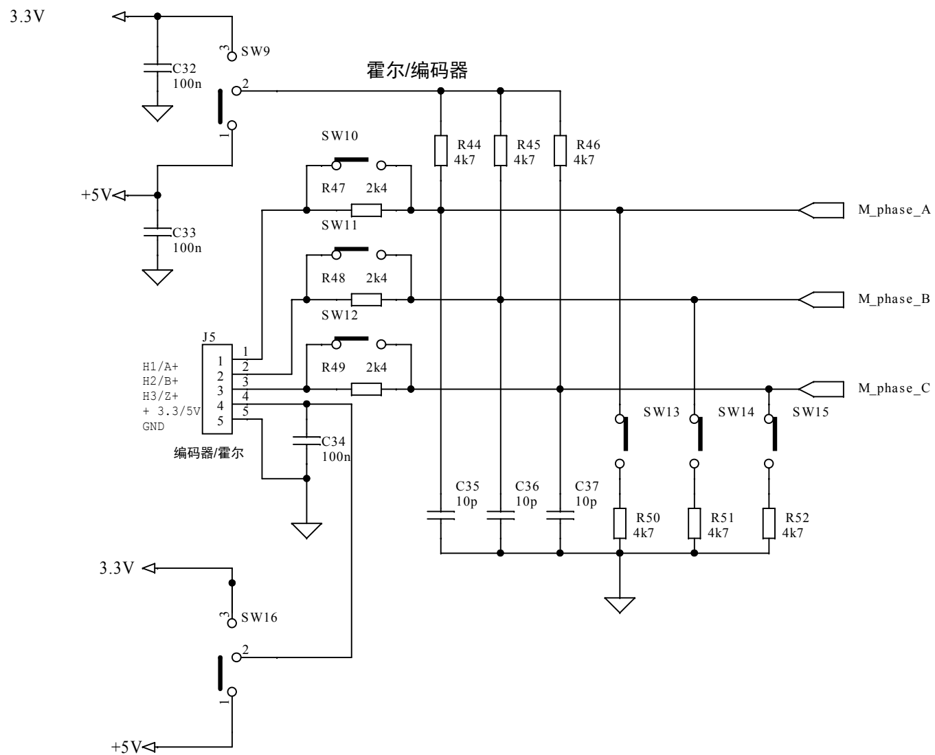
图 5. STEVAL-IPM20B 板原理图 (图 5, 共 5 图)
