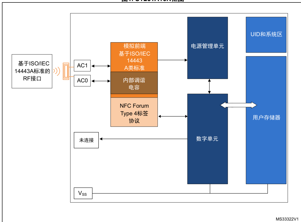
图1. ST25TA16K框图
