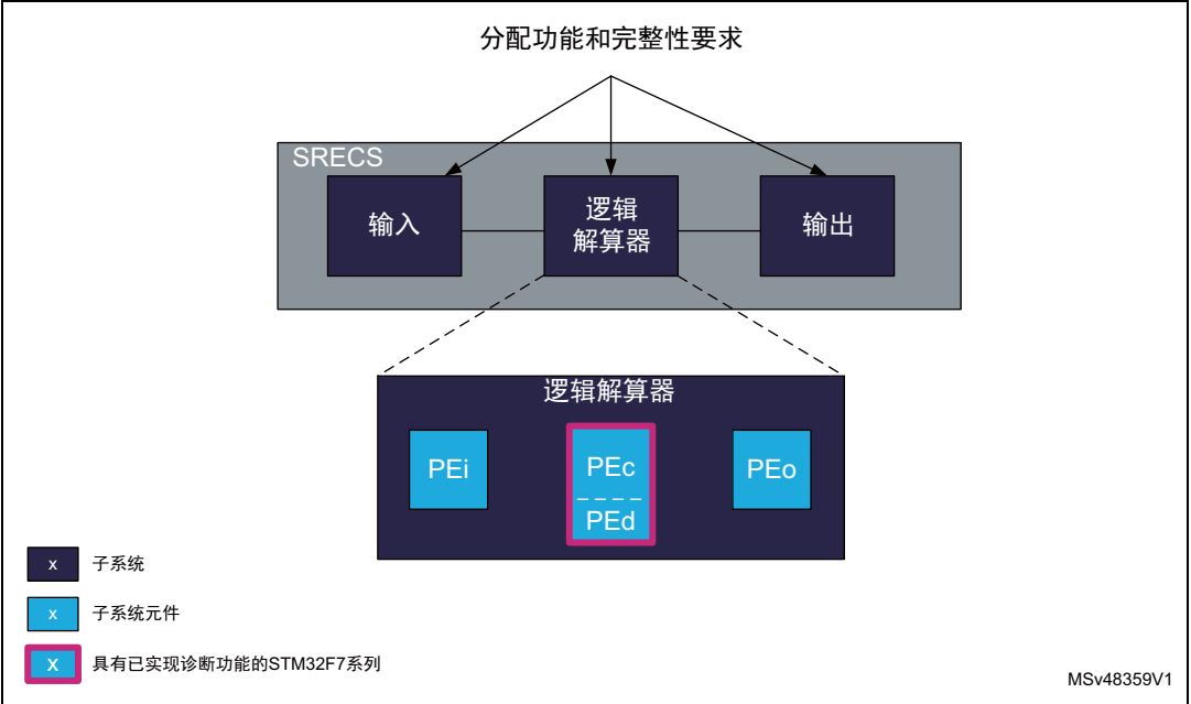
图9. SRECS高层图
