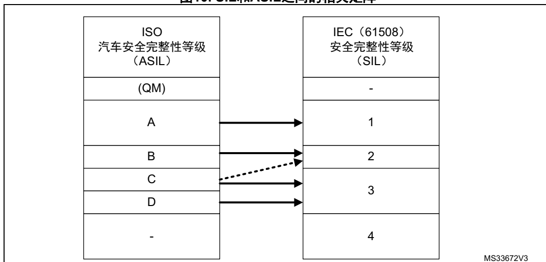
图10. SIL和ASIL之间的相关矩阵
